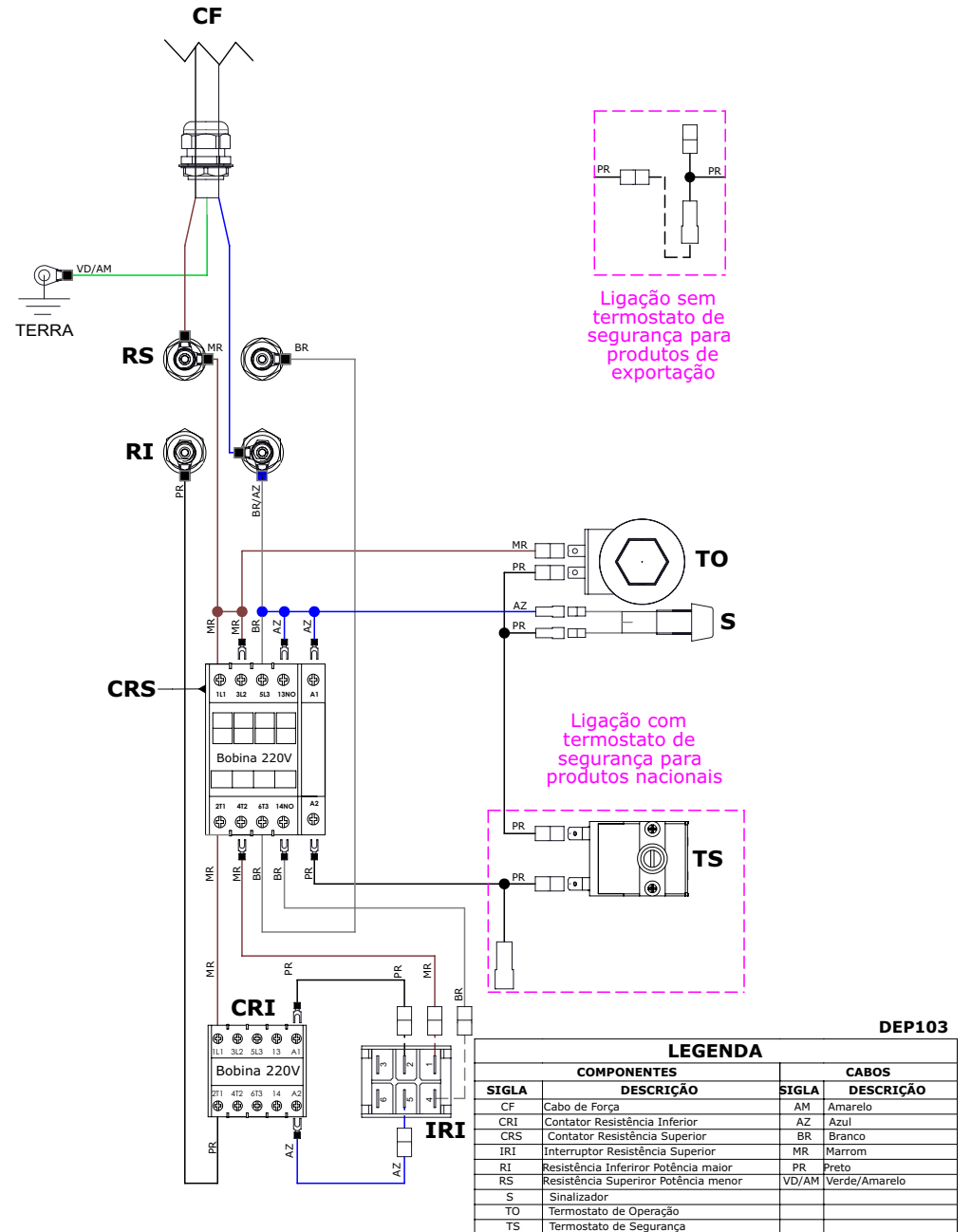
DIAGRAMA ELÉTRICO DO MODELO PR-30 R (220V):
